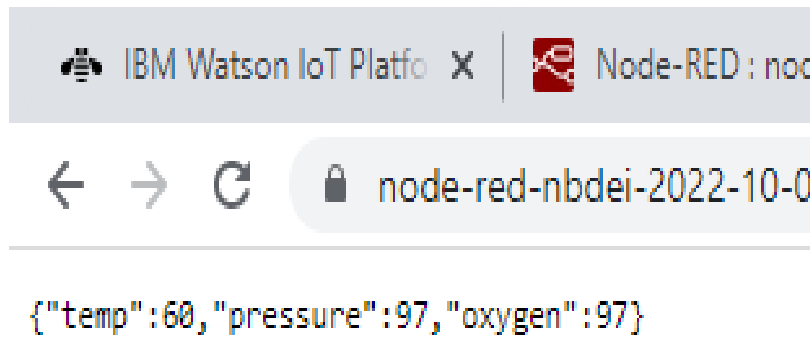
Fig 3. Browser Output
