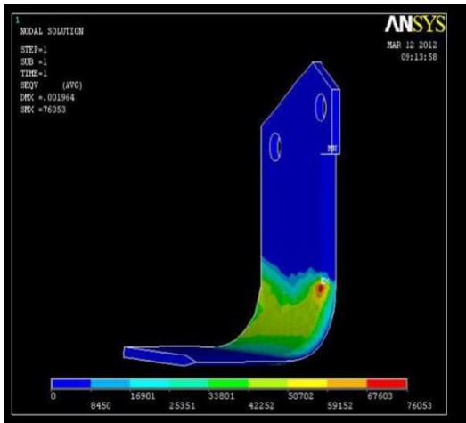
Fig 11: Die Steel
