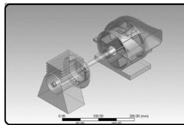
Fig. 2. Centrifugal blower
